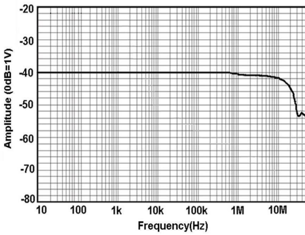
图 4 CP6150 幅频曲线
