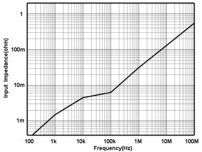
图 3.b CP6030A 输入阻抗 VS 频率曲线
