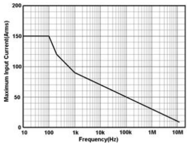
图 5 CP6150 最大测量电流 VS 频率曲线
