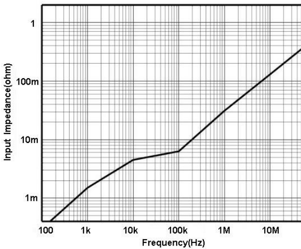
图 3.a CP6030 输入阻抗 VS 频率曲线
