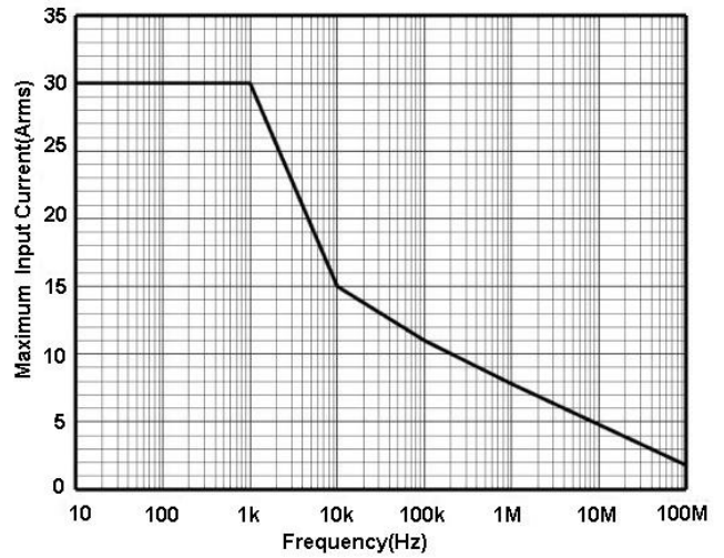
图 2.b CP6030A 最大测量电流 VS 频率曲线
