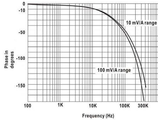
CP4070A 1A 峰值时典型的相位与频率对应图
