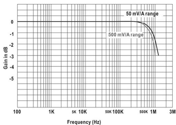
CP4050 1A 峰值时典型的增益频率对应图
