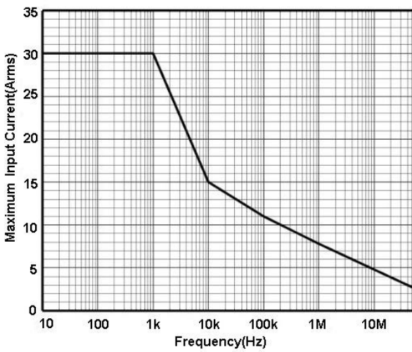
图 2.a CP6030 最大测量电流 VS 频率曲线
