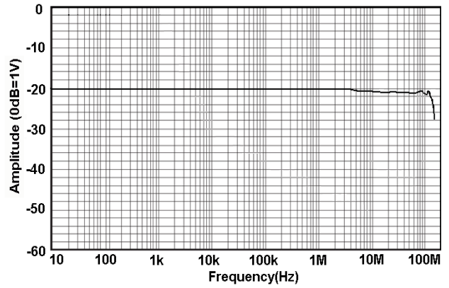
图 1 .b CP6030A 幅频曲线
