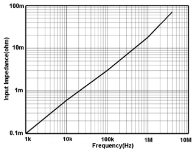
图 9 CP6500 输入阻抗 VS 频率曲线
