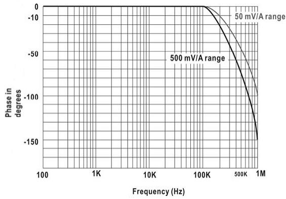
CP4050 1A 峰值时典型的相位与频率对应图
