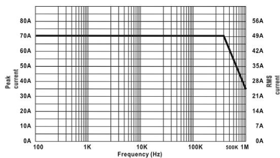
CP4050 最高电流量与频率对应图
