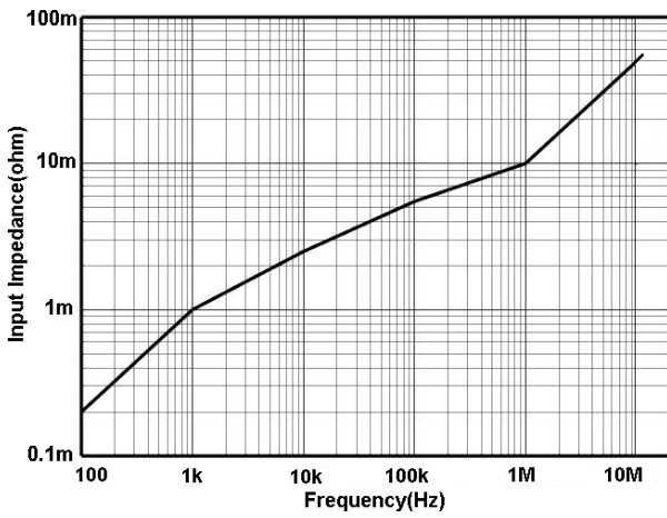
图 6 CP6150 输入阻抗 VS 频率曲线
