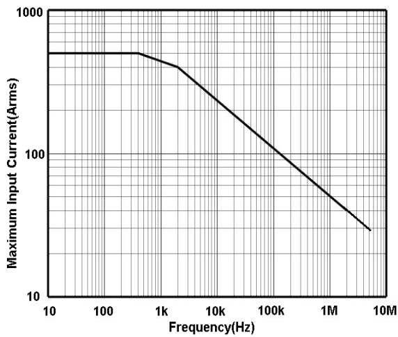
图 8 CP6500 最大测量电流 VS 频率曲线
