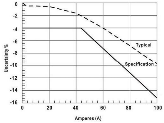
CP4070A 10mV/A 时典型的 DC 信号线性
