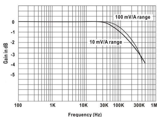
CP4070A 1A 峰值时典型的增益频率对应图
