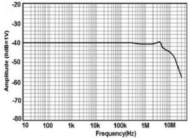
图 7 CP6500 幅频曲线
