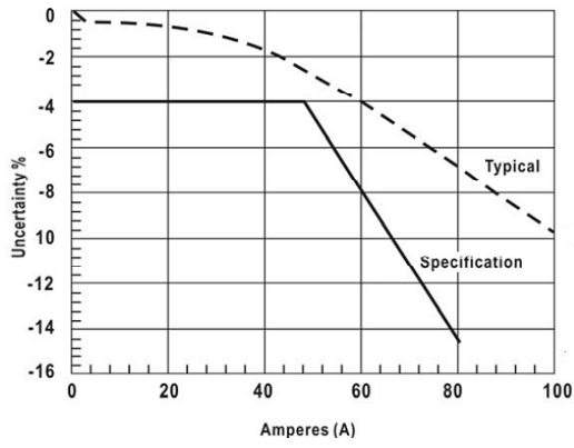
CP4050 50mV/A 时典型的 DC 信号线性
