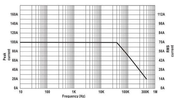
CP4070A 最高电流量与频率对应图
