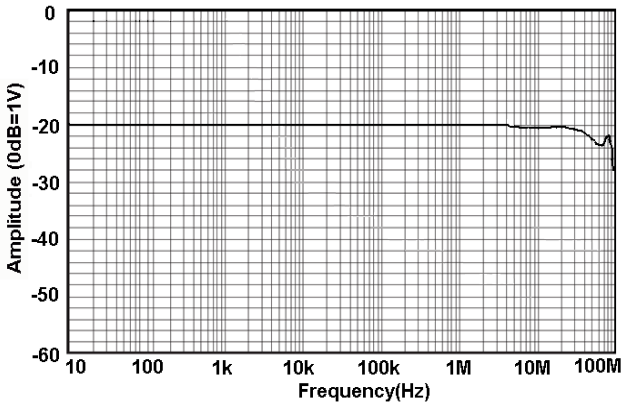
图 1 .a CP6030 幅频曲线
